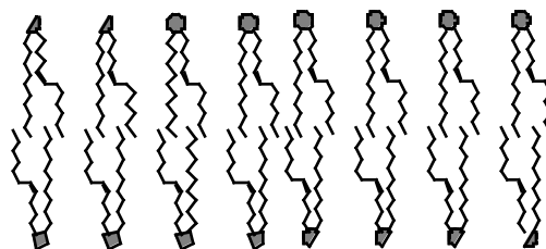
membrane bilayer
