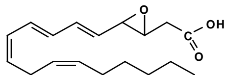
LEUKOTRIENE A
