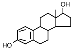
ESTRADIOL
