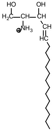
SPHINGOSINE
